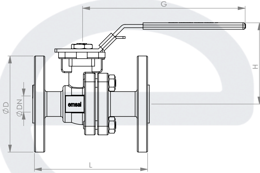
ÖLÇÜLER / DIMENSIONS
